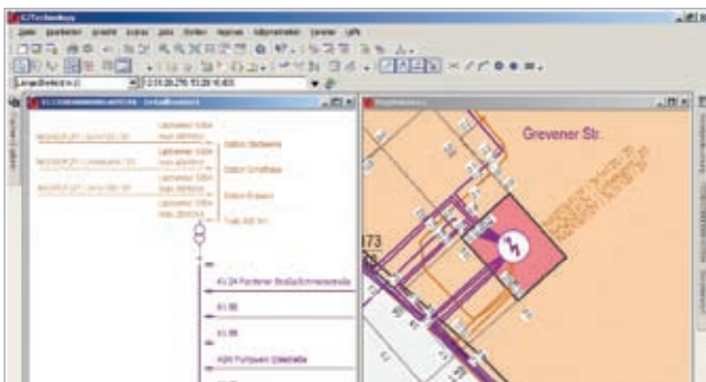
Bestandsplan mit Trafostation und Detailfenster mit dem Innenleben dieser Trafostation
