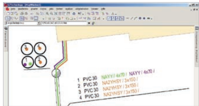
Querschnitt Leitungskanal mit Schutzrohrpaket
